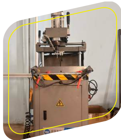
Máý phay chép hình (High-speed copy milling machine)
